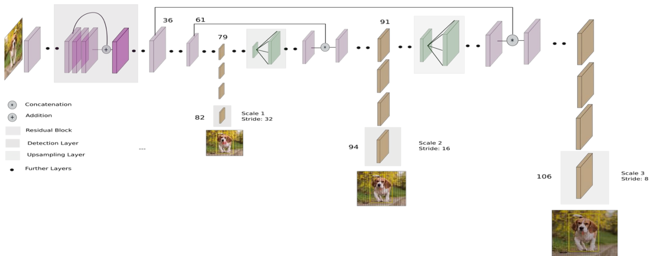
Ilustración 5. Arquitectura YOLO
